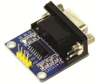
MAX 232 TO TTL
